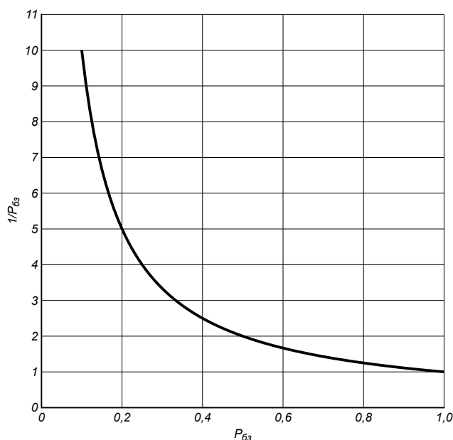
Рисунок 5 – Зависимость 1/P_{б3}
