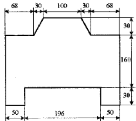
Боевая машина пехоты (мишень №14)
