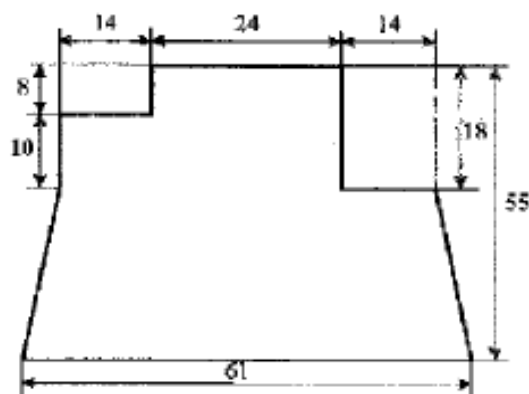
Поясная фигура (мишень №7б)
